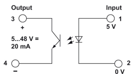
Schaltsymbol
