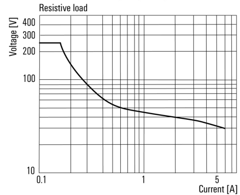
Curva de límite de carga DC
