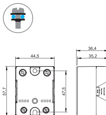
Tipo 77.x5 Bornes a pletina
