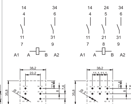
62.22- 4300 Vista parte inferior
