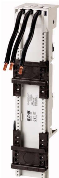
Busbar adapter, 55 mm, 63 A, DIN rail: 2
