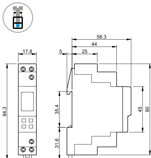
Tipo 12.71 Borne de jaula
