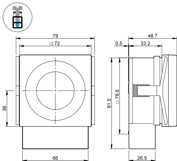
Tipo 12.71 Borne de jaula
