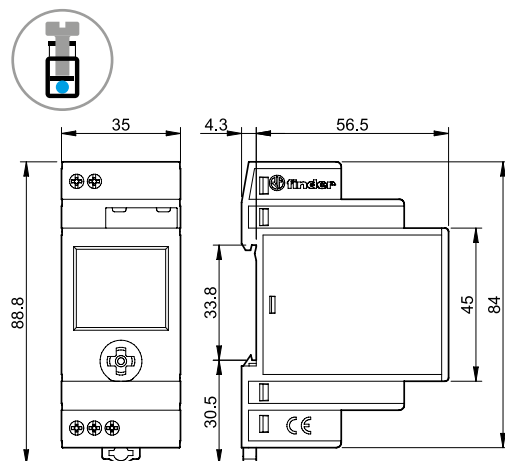
Tipo 12.51/12.81 Borne de jaula
