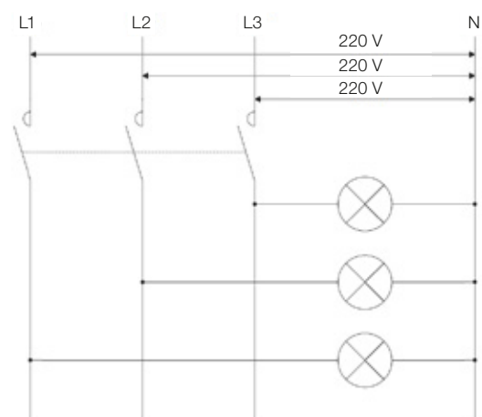
Circuito trifásico conectado en estrella
