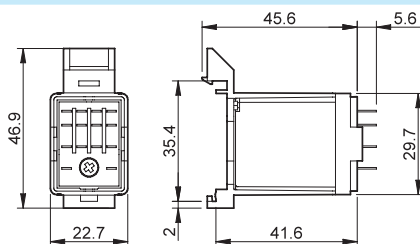
056.27 con relé
