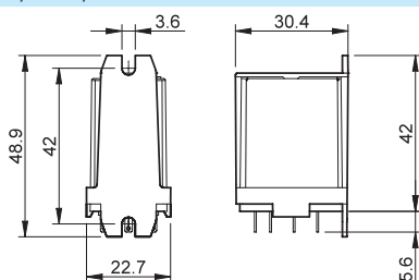
056.26 con relé
