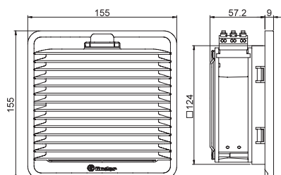
Tipo 7F.xx.x.xxx.2055 Bornes Push-in
