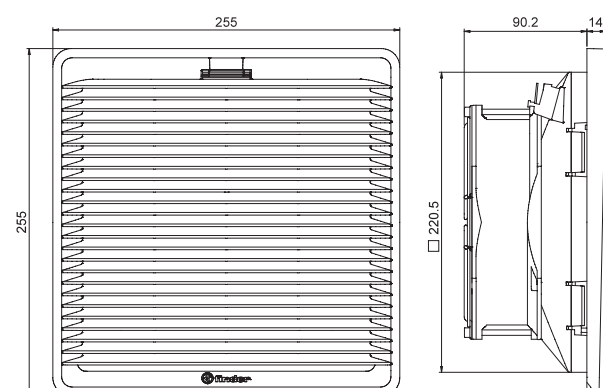
Tipo 7F.xx.x.xxx.4250 Bornes Push-in
