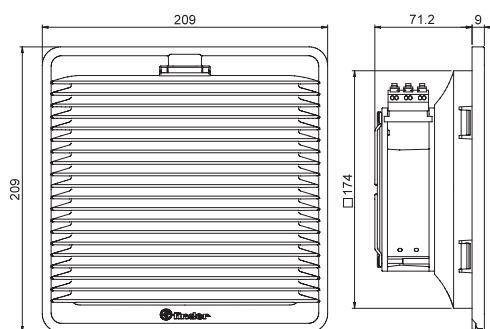
Tipo 7F.xx.x.xxx.3100 Bornes Push-in
