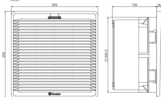
Tipo 7F.xx.x.xxx.4400 Bornes Push-in
