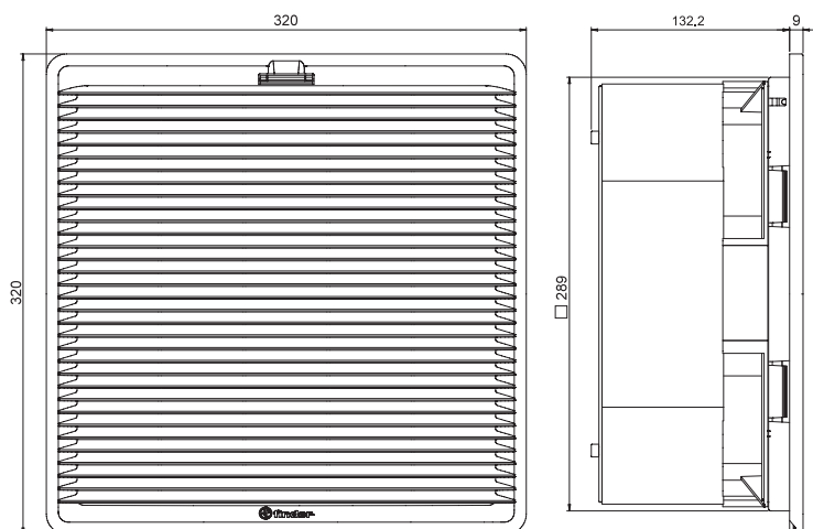
Tipo 7F.xx.x.xxx.5700 Bornes Push-in
