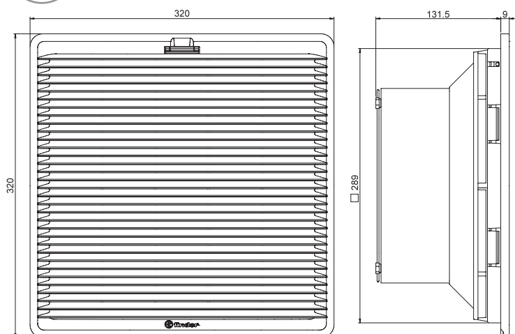
Tipo 7F.xx.x.xxx.5550 Bornes Push-in
